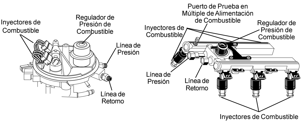
Cuerpo del Estrangulador (CFI) de Ford
