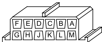
DLC del ALDL
